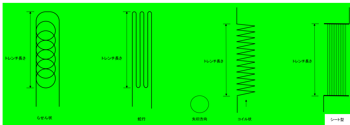
図 0.2 水平埋設型の場合の熱交換器長 L_{exch,i}
