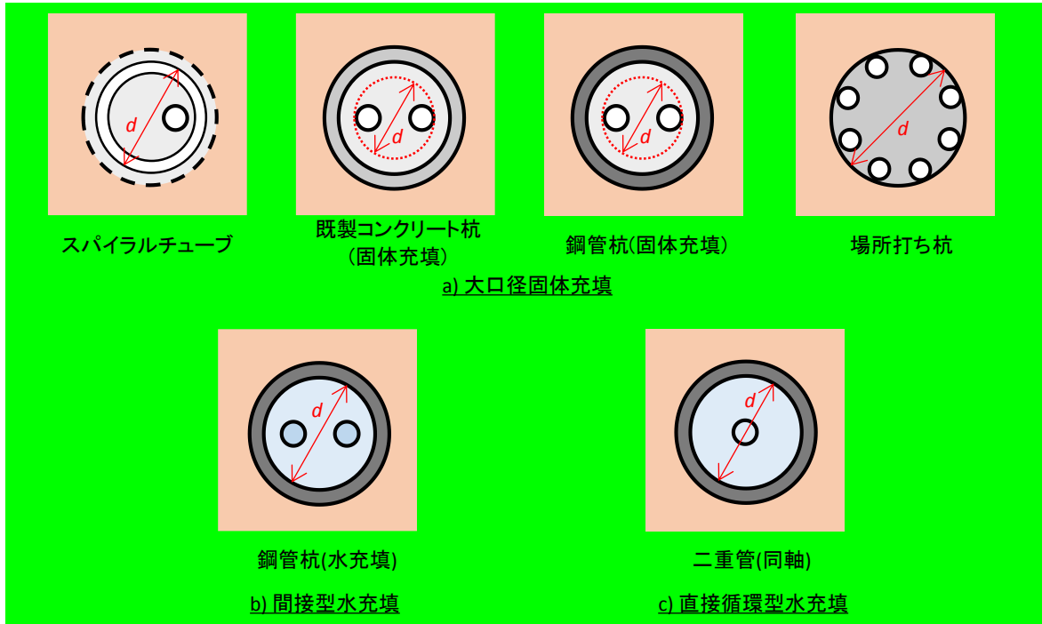
図 0.3 熱交換器の断面の直径に係る寸法 d_{exch,i} (特定非営利活動法人地中熱利用促進協会資料をもとに作成)
