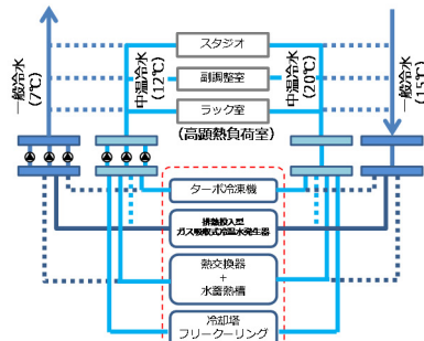
熱源（中温冷水による高COP運転）
