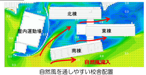
自然風を通しやすい校舎配置
