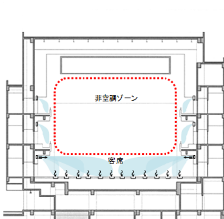
壁吹出・床吸込の気流イメージ
