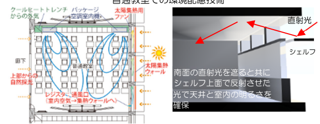
ライトシェルフによる自然光導入
