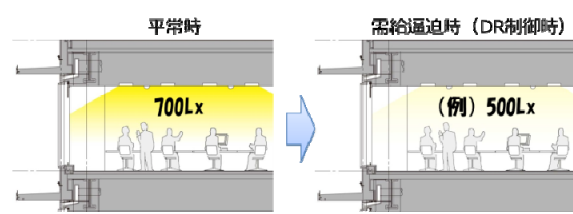
〈照明出力抑制制御〉
