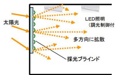
事務室ゾーンにおける自然光利用
