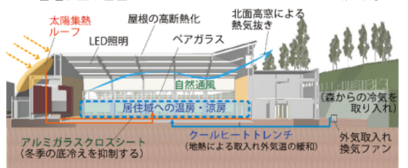
屋内運動場での環境配慮技術
