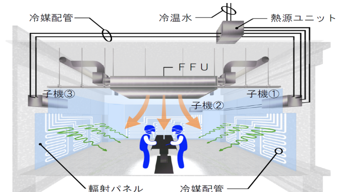
手術室輻射空調概念図
