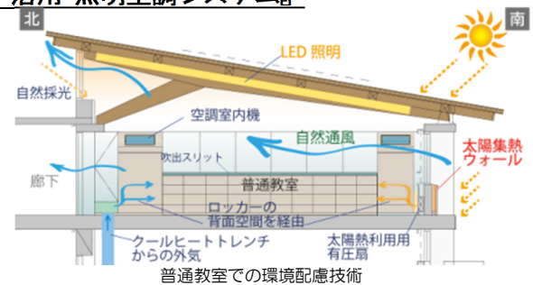
普通教室での環境配慮技術
